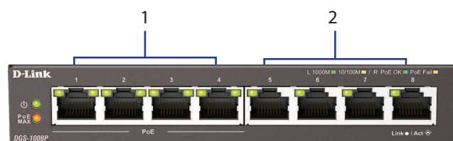
Afbeelding 2: aansluitingen op het voorpaneel
