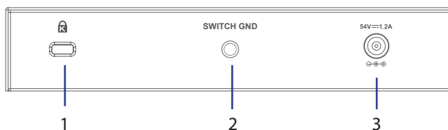
Bild 3: Anslutningar bakre panel
