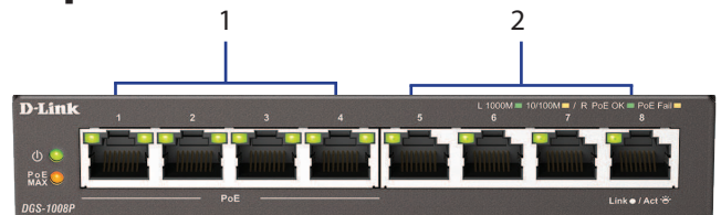
Kuva 2: Etupaneelin liittimet
