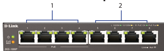
2. ábra: Csatlakozók az elülső panelen
