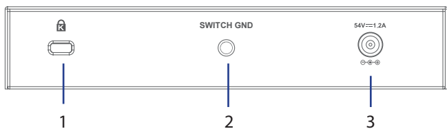
Figura 3: Conectores do painel traseiro
