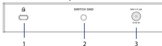
Obrázek 3: Zadní konektory
