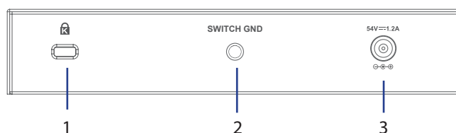
Figura 3: Connettori pannello posteriore
