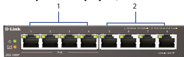
Εικόνα 2: Σύνδεσμοι στο εμπρός πάνελ
