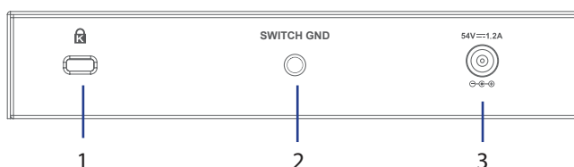
3. ábra: Csatlakozók a hátsó panelen
