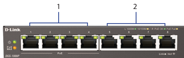
Figura 2: Connettori pannello frontale
