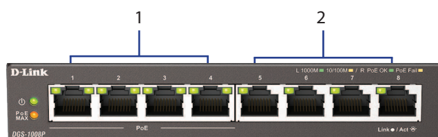
Rysunek 2: Złącza na panelu przednim
