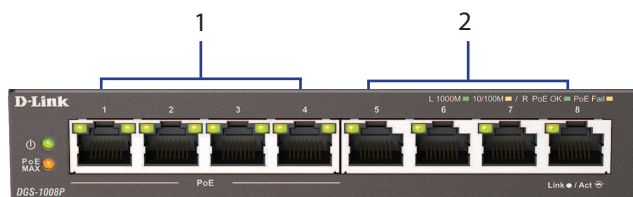
Obrázek 2: Přední konektory
