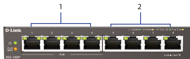
Figur 2: Stik på frontpanelet
