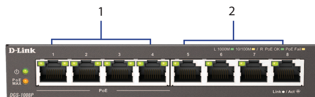
Slika 2: Priključci na prednjoj ploči
