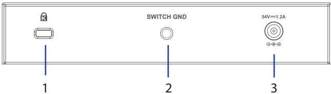
Figure 3 : Connecteurs du panneau arrière
