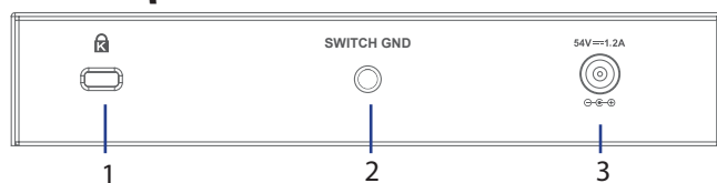
Εικόνα 3: Σύνδεσμοι στο πίσω πάνελ
