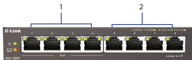
Figura 2: Conectori panou frontal
