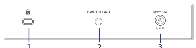
Kuva 3: Takapaneelin liittimet
