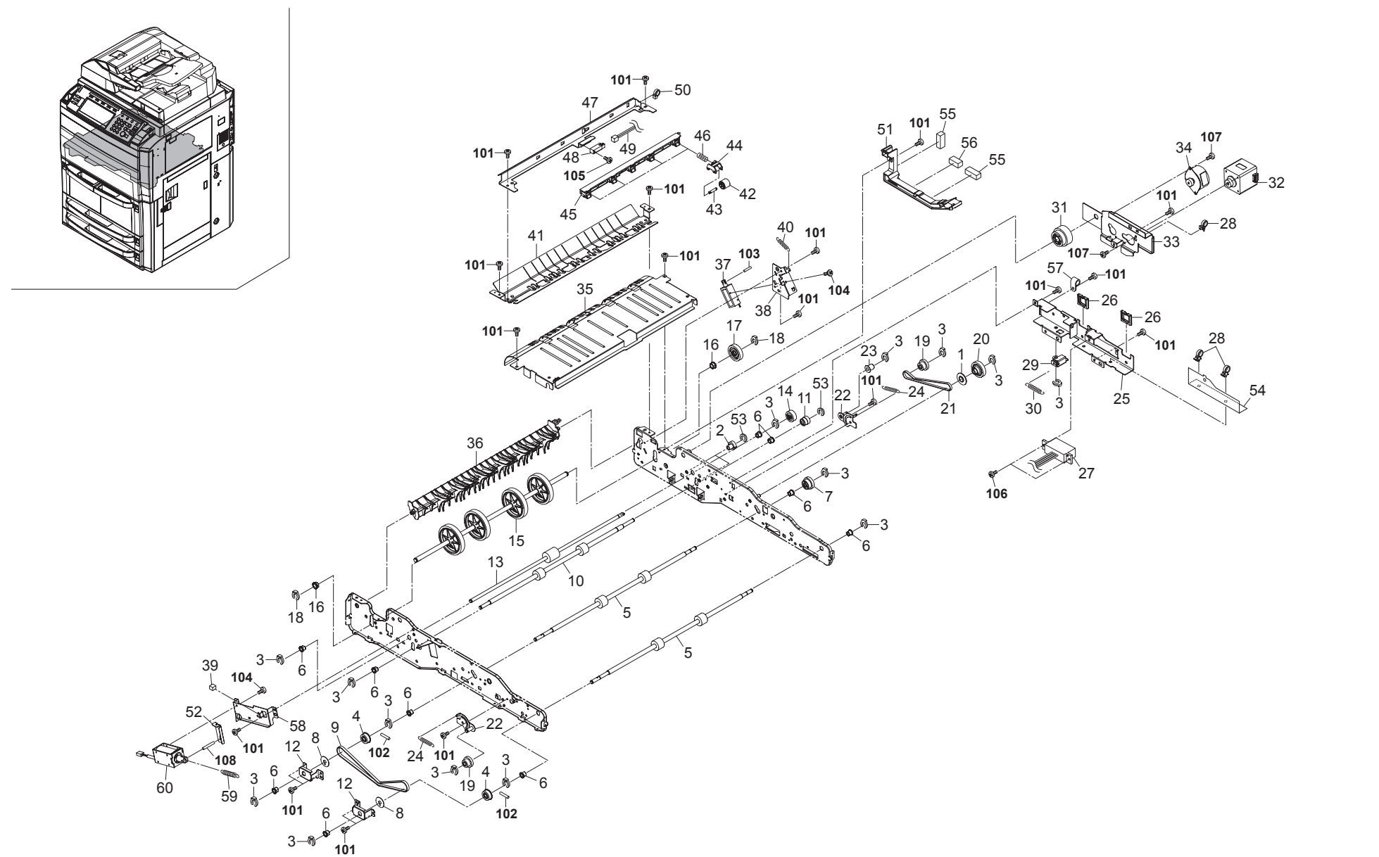
FIG. 27 Duplex Section 2
