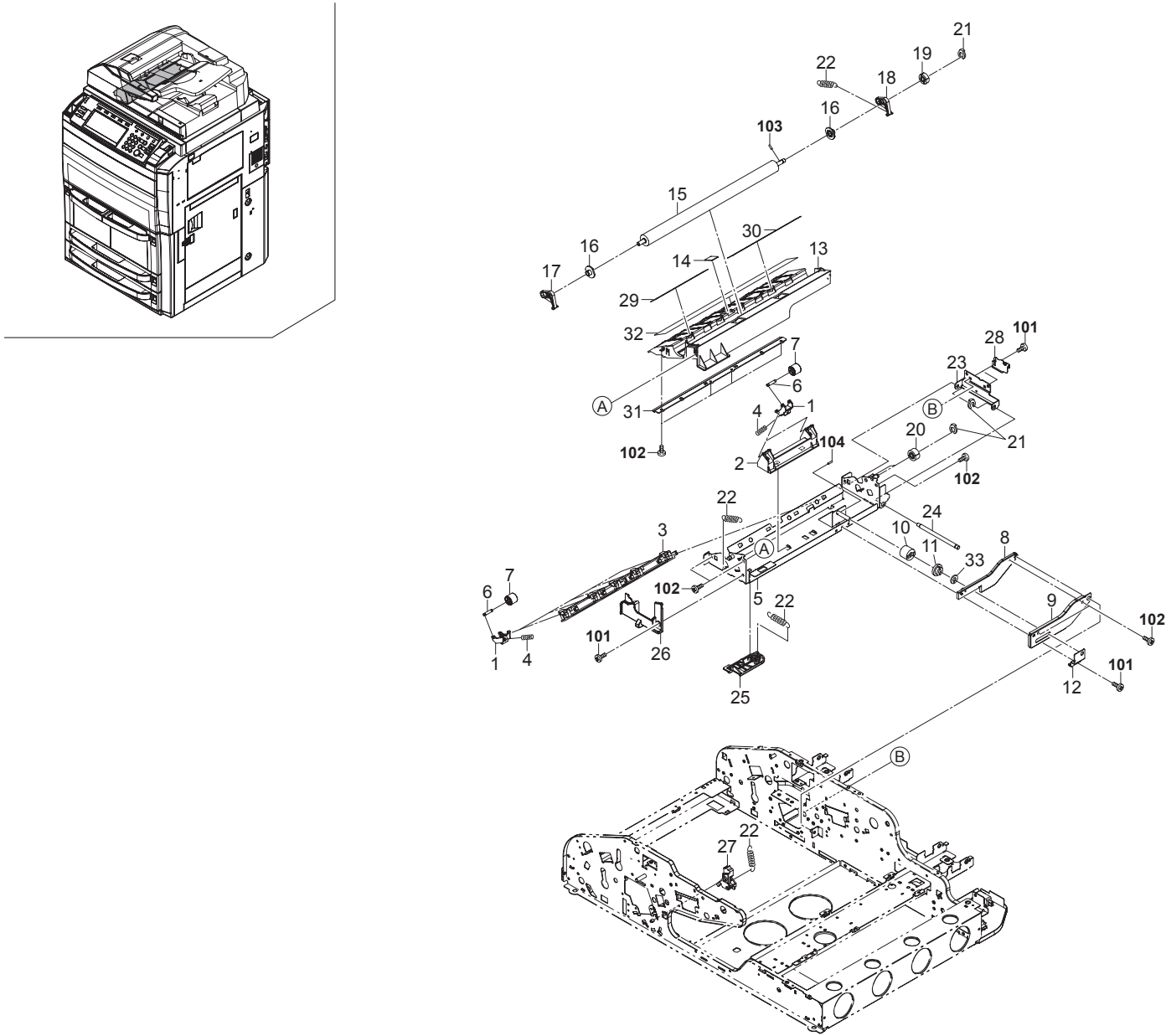
FIG. 38 Duplex Section (DP)
