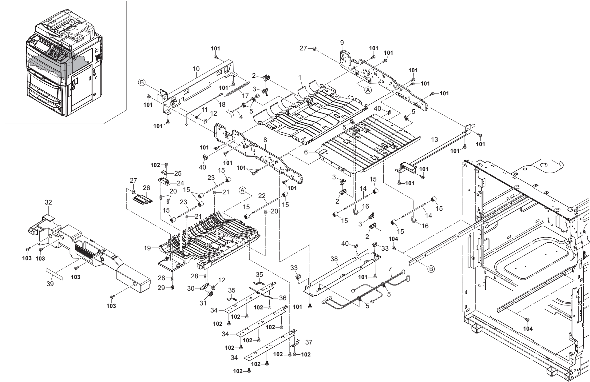
FIG. 26 Duplex Section 1
