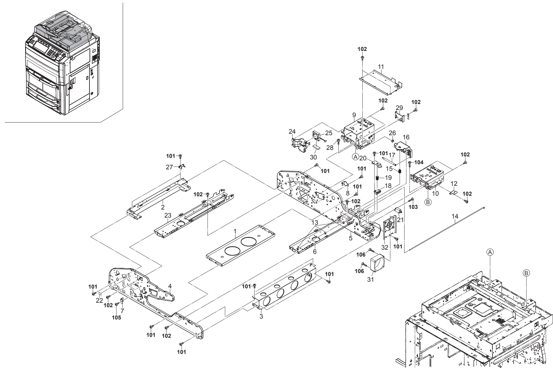
FIG. 35 Frames (DP)
