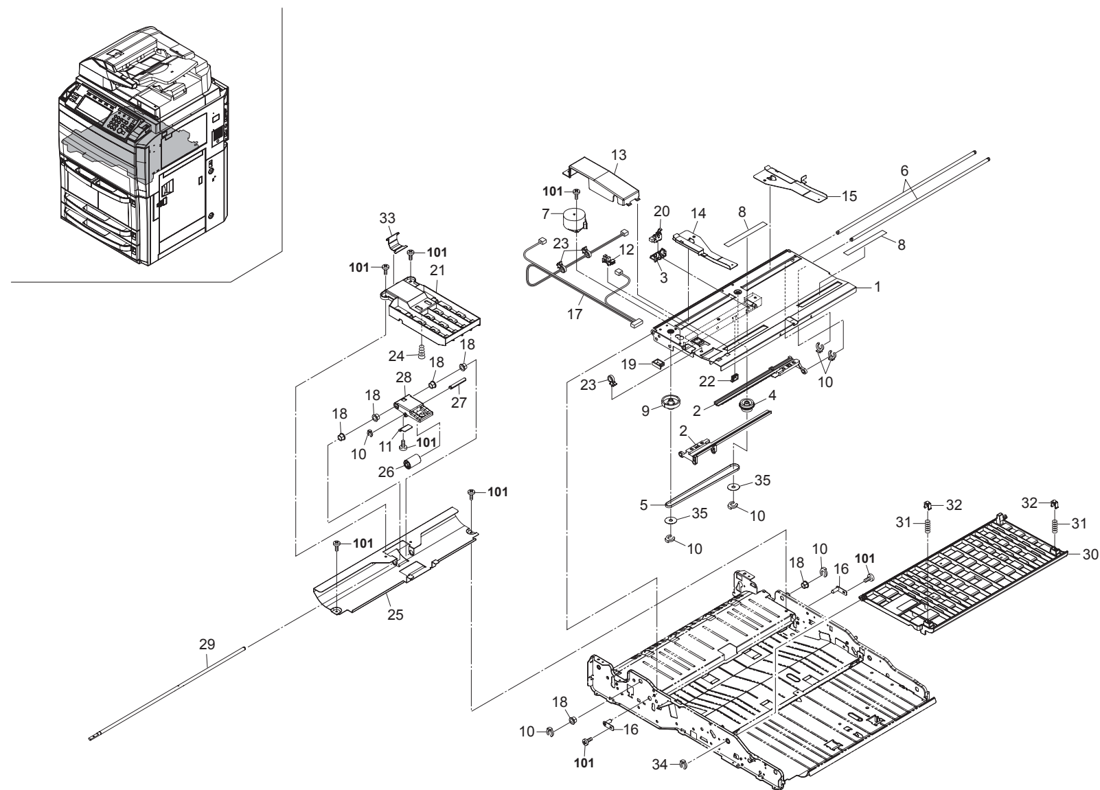
FIG. 28 Duplex Section 3
