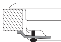
Posición del gancho para superficies H=30mm
