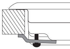
Position der Haken für Arbeitsplatten H=30mm
