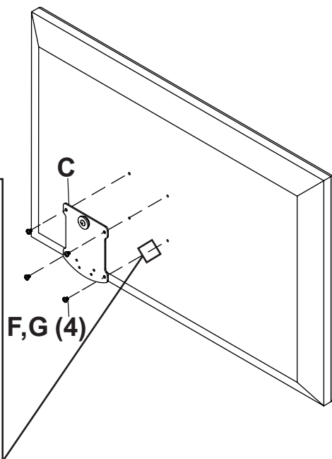
VESA 200:
