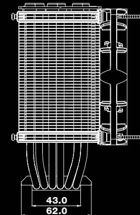
ANSICHT LINKE SEITE ▼ LEFT SIDE ▼
