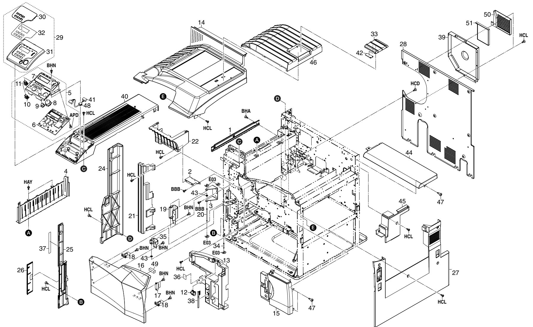
FIG. 1 Enclosure
