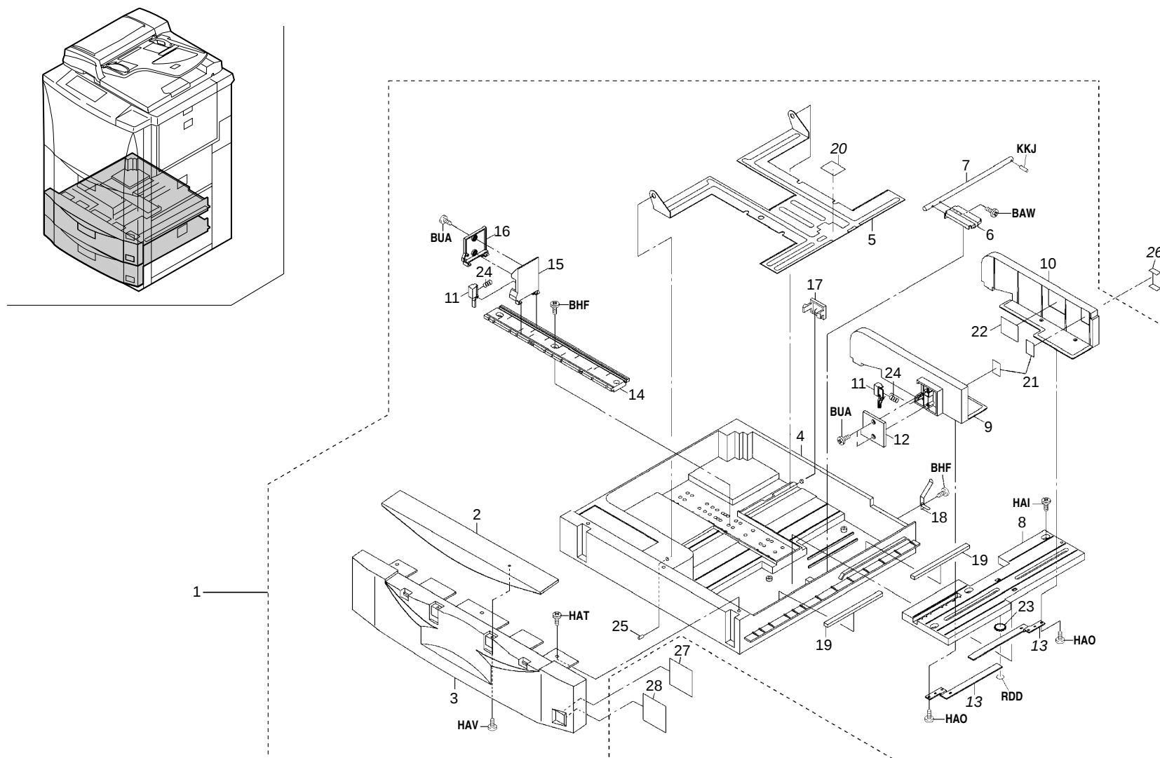
FIG. 3 CASSETTE(230/240V)
