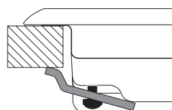
Stand haak voor keukenblad H=20mm
