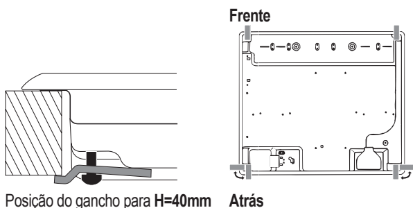
Posição do gancho para H=40mm
