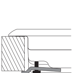
Position der Haken für Arbeitsplatten H=40mm
