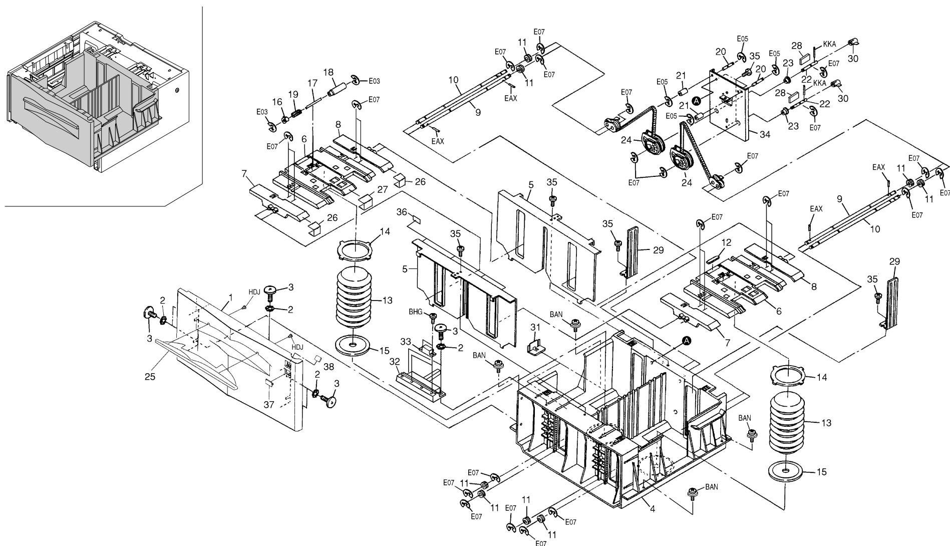
FIG. 2 CASSETTE
