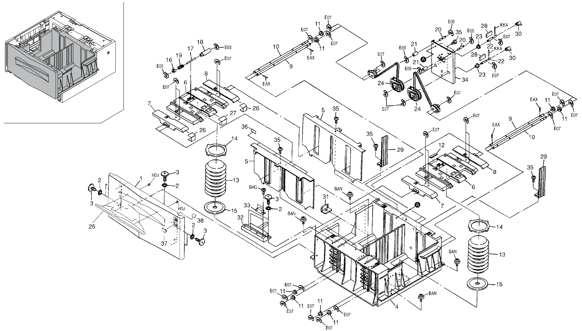
FIG. 2 CASSETTE
