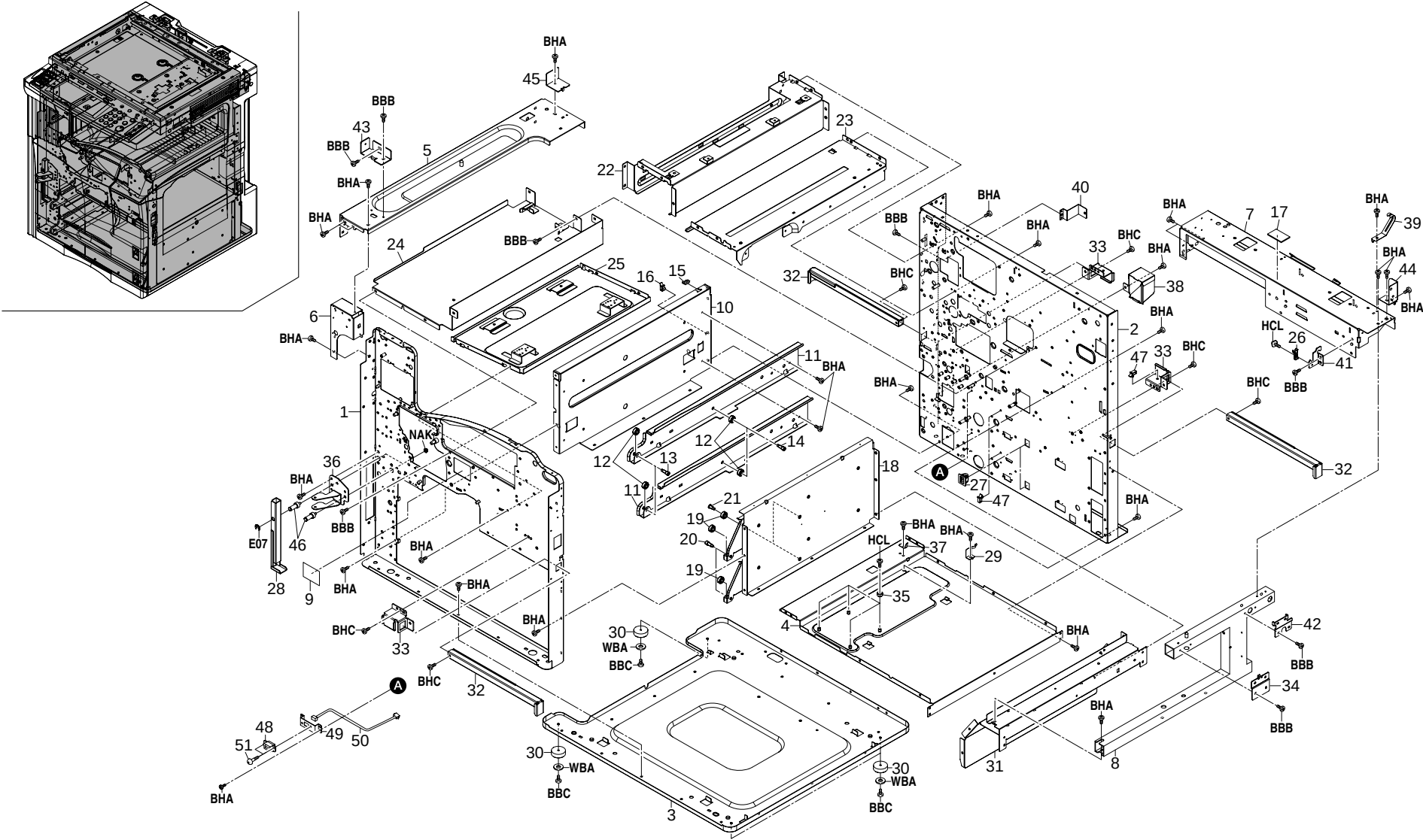
FIG. 2 FRAMES
