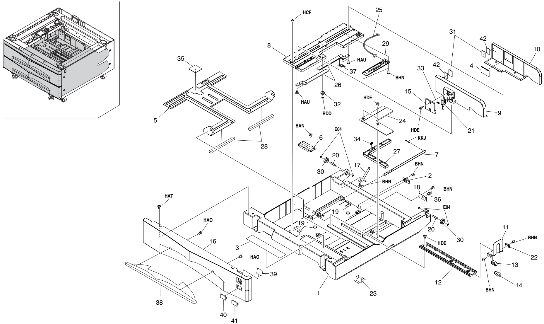
FIG. 3 CASSETTE
