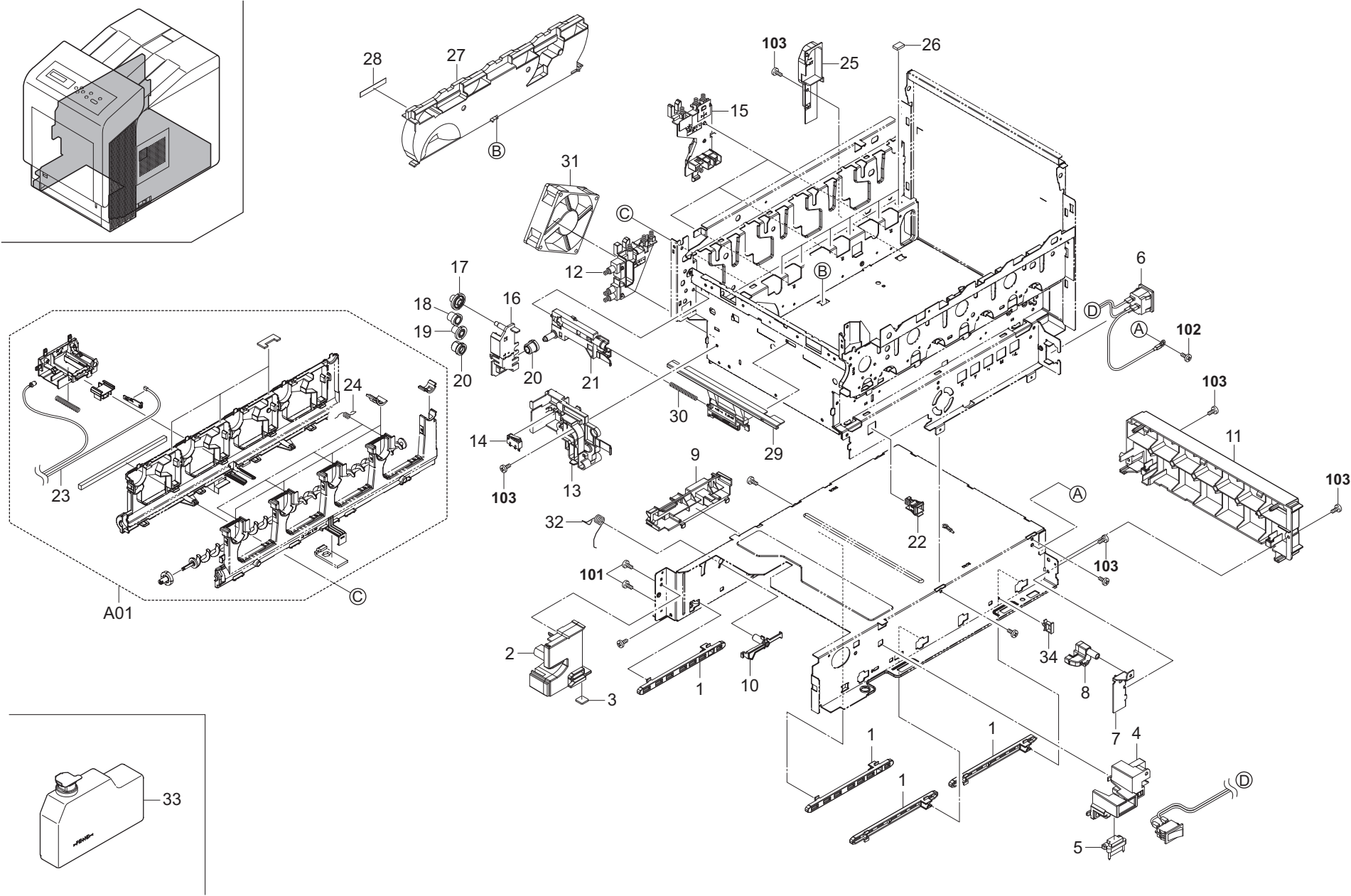
FIG. 4 Frames 2
