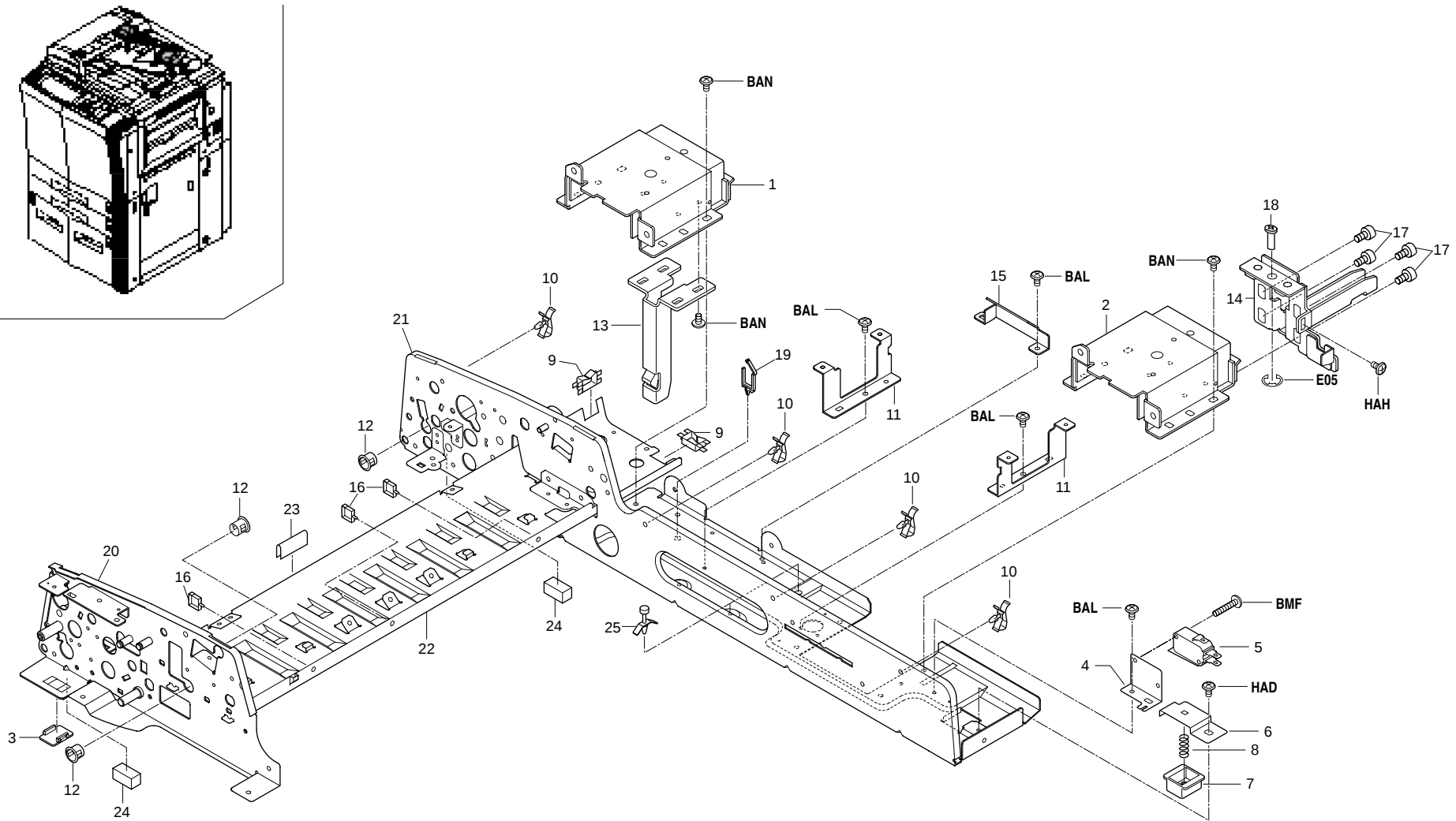
FIG. 32 FRAME SECTION (DF)
