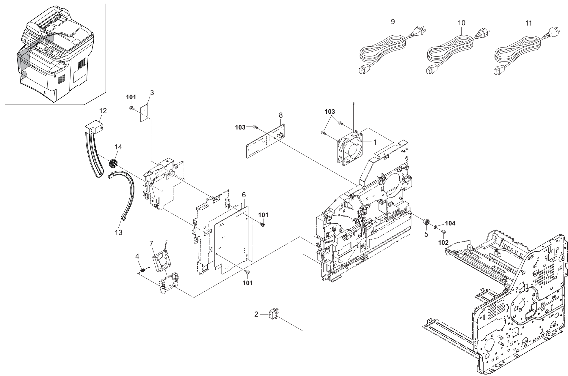
FIG. 3 Frames 2
