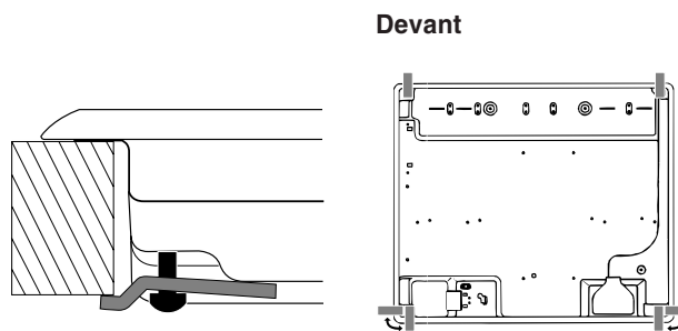
Position du crochet pour plan H=40mm
