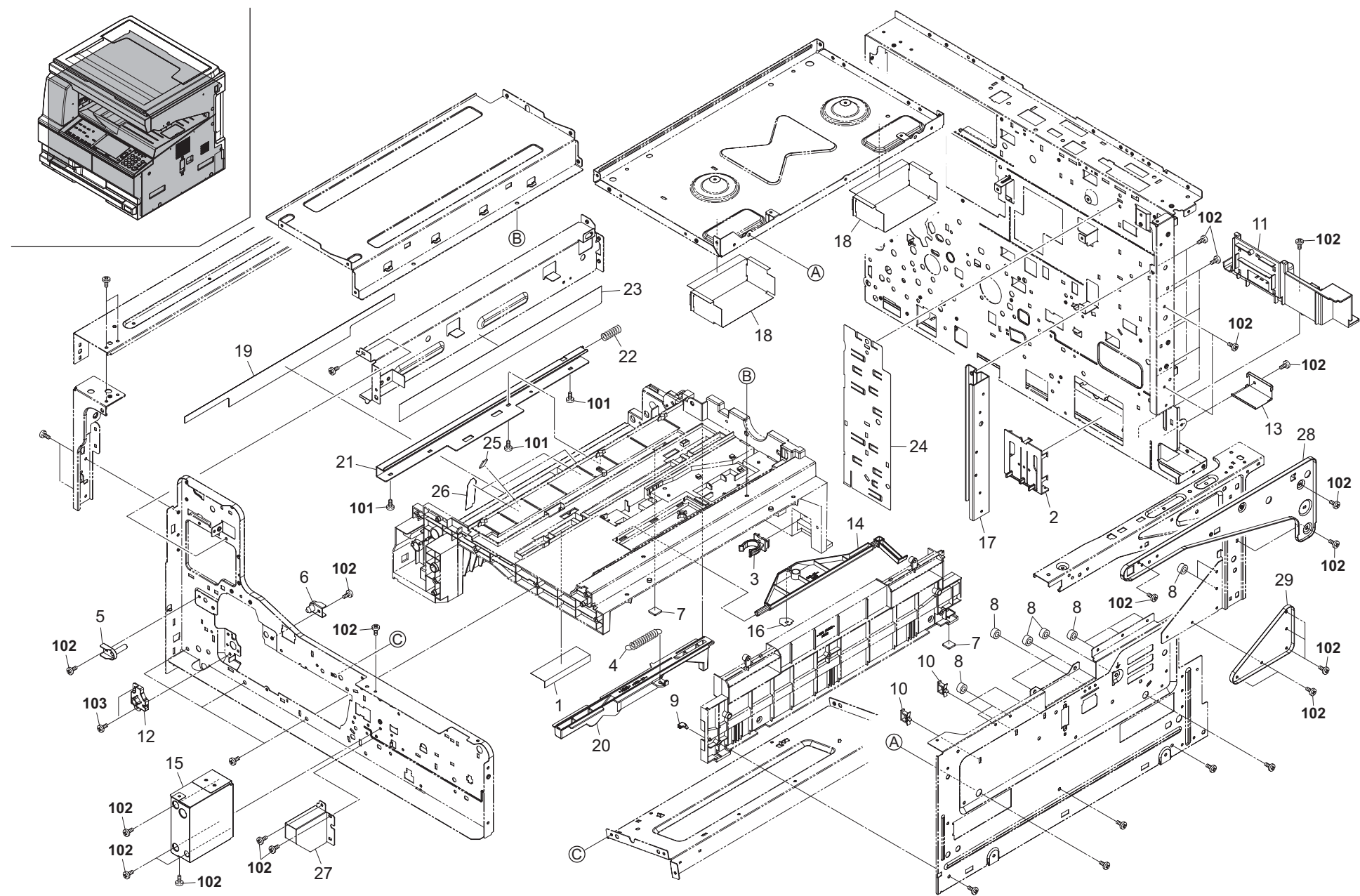
FIG. 2 Frames 1
