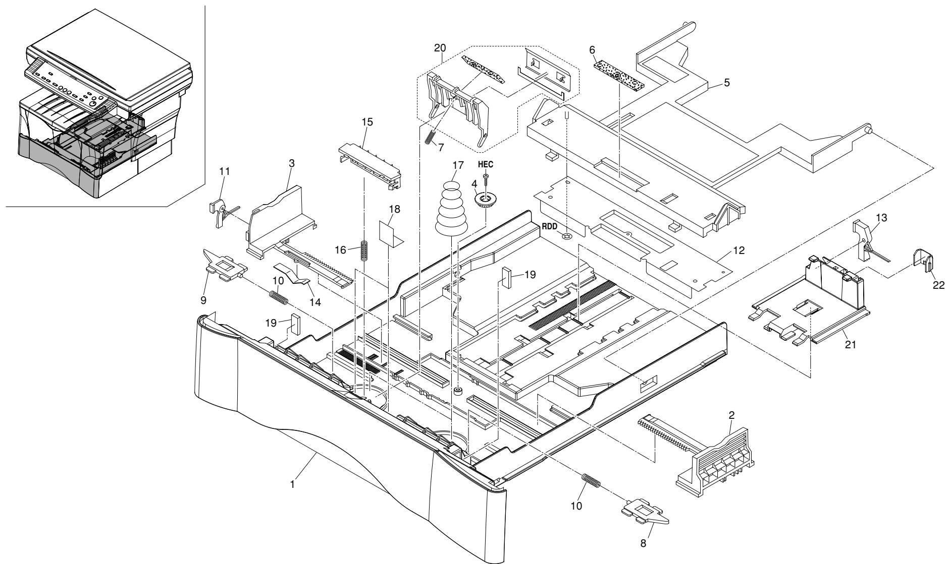
FIG. 7 CASSETTE
