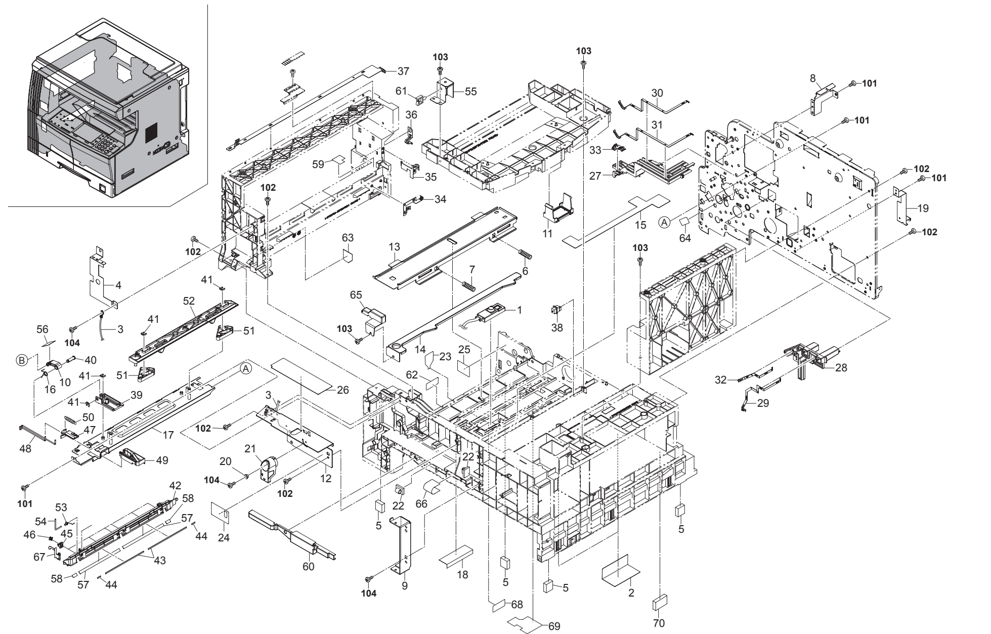
FIG. 2 Frames
