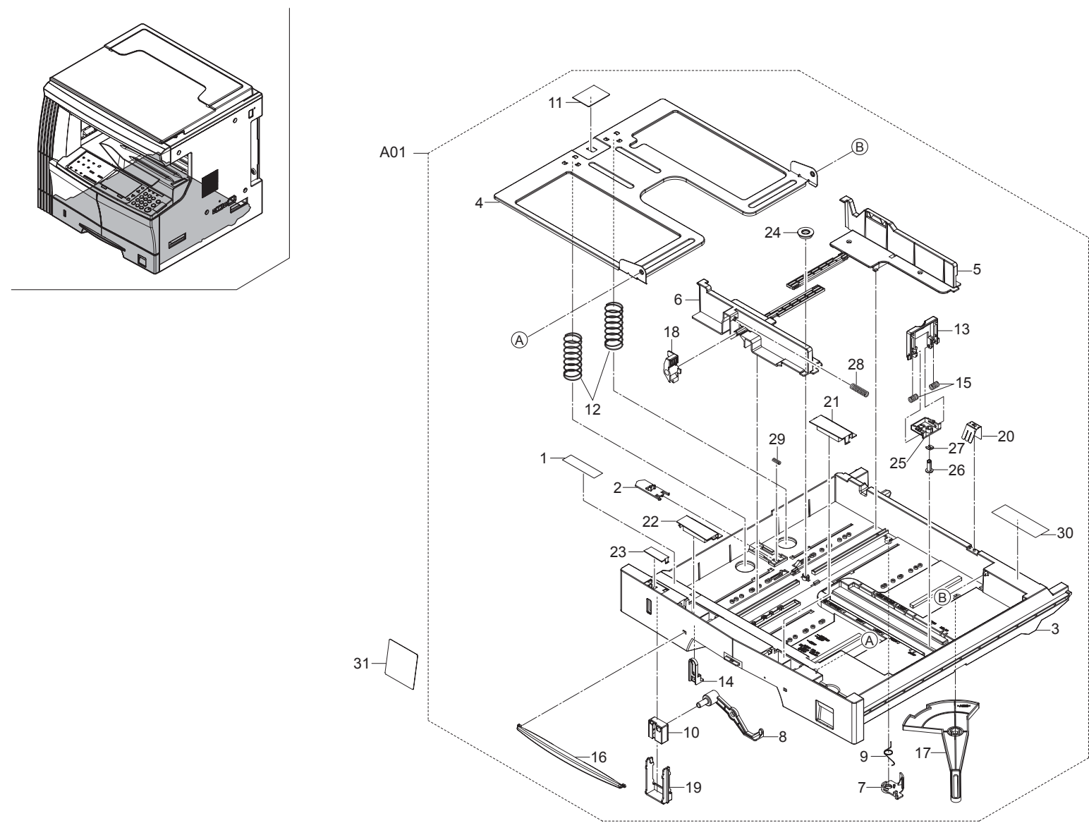
FIG. 3 Cassette
