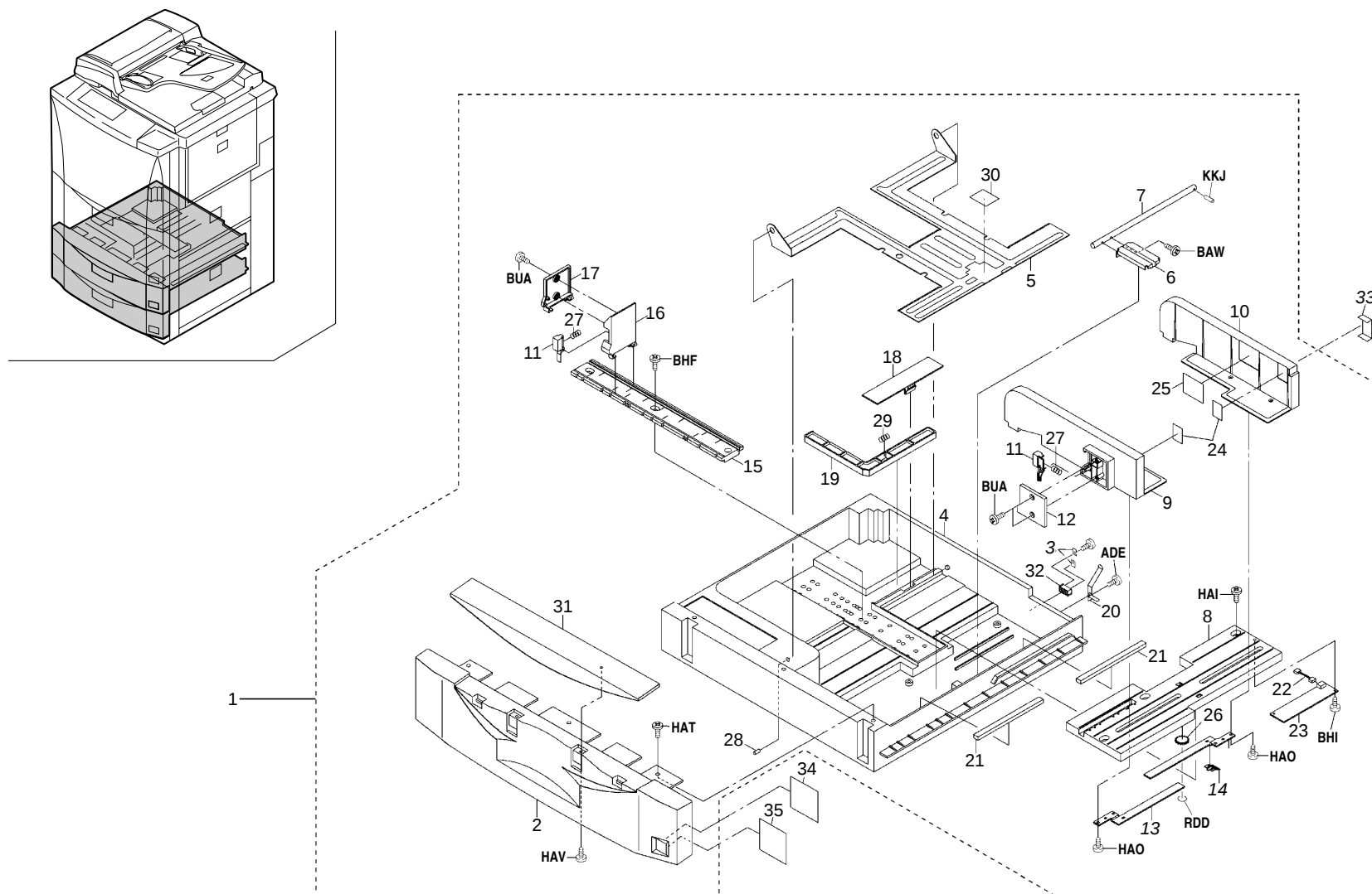
FIG. 3 CASSETTE(120V)
