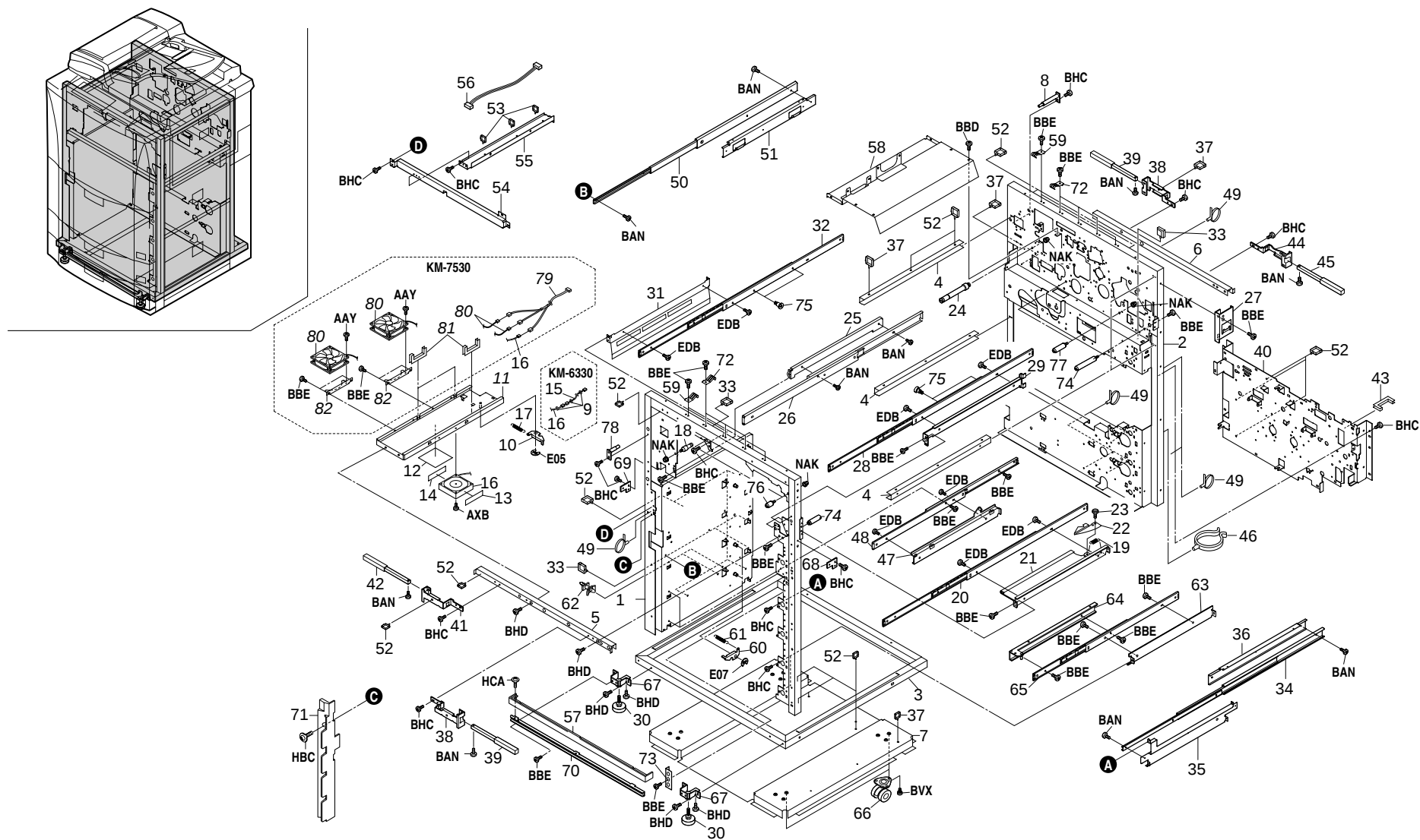
FIG. 2 FRAMES
