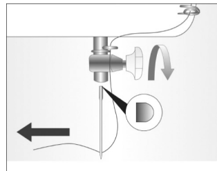
Estrazione dell'ago
