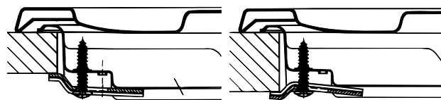
Position du crochet pour plan H=20mm
