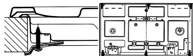
Position du crochet pour plan H=40mm
