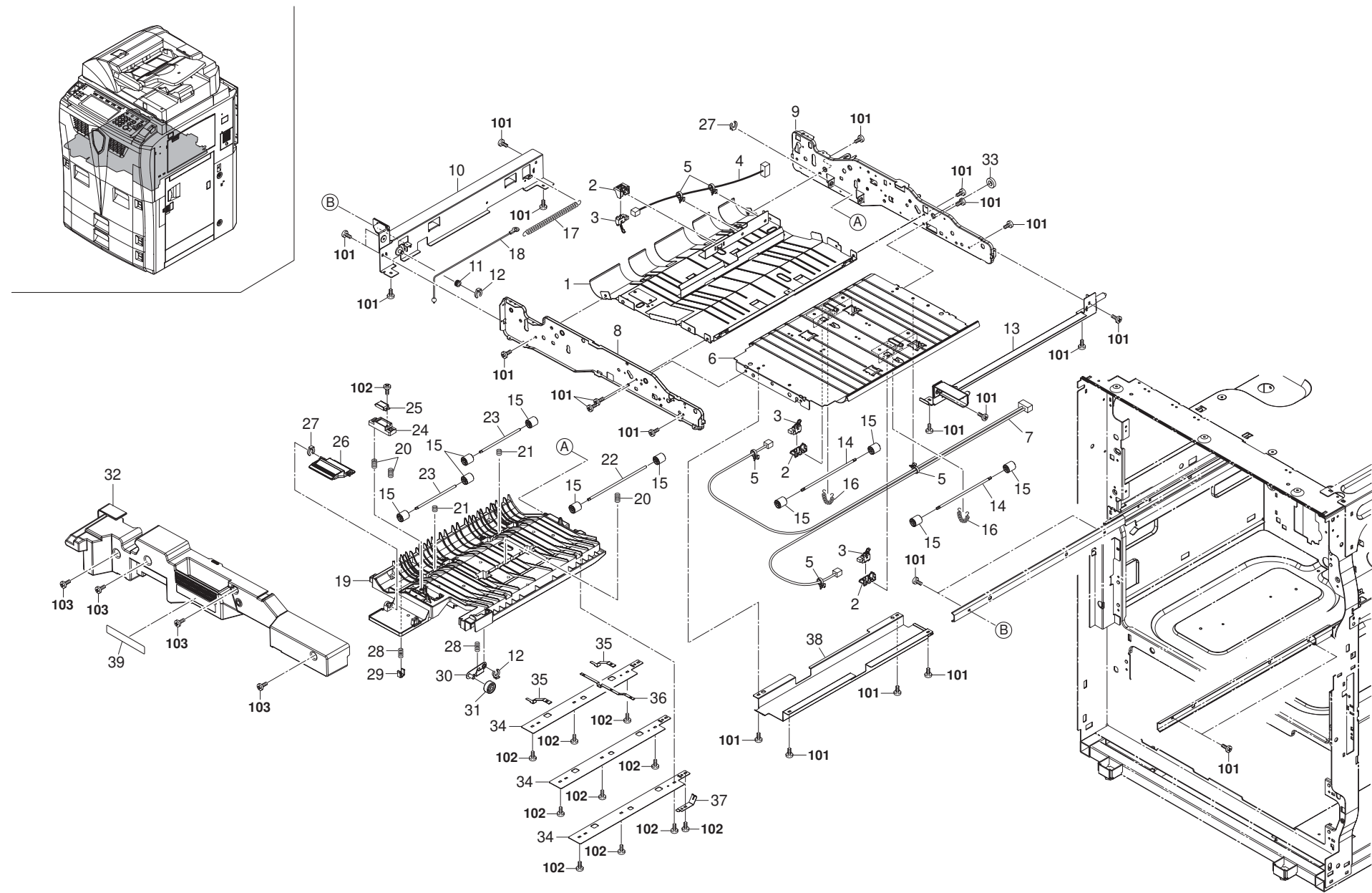
FIG. 26 Duplex Unit I
