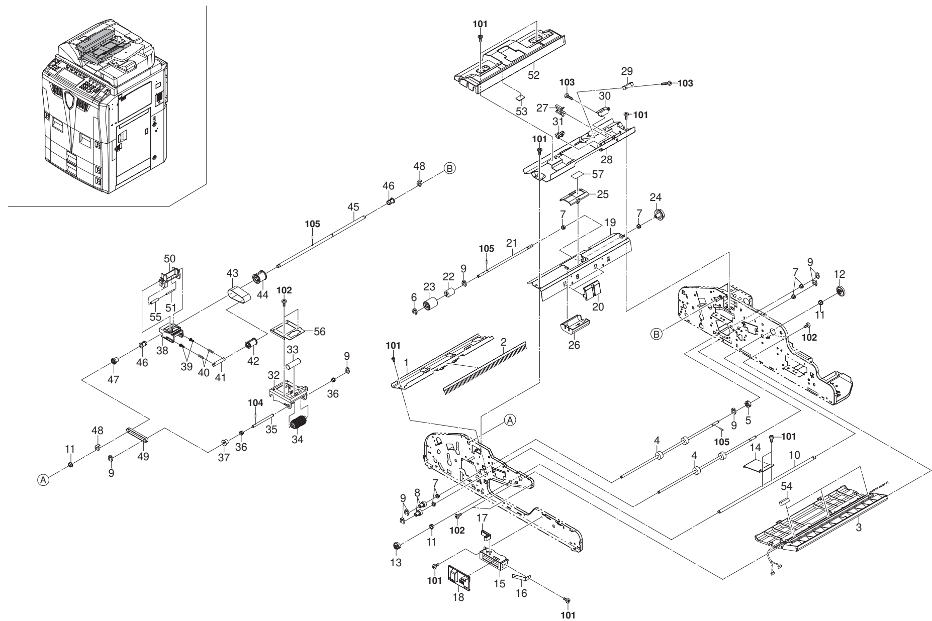
FIG. 39 Paper Eject (DP)
