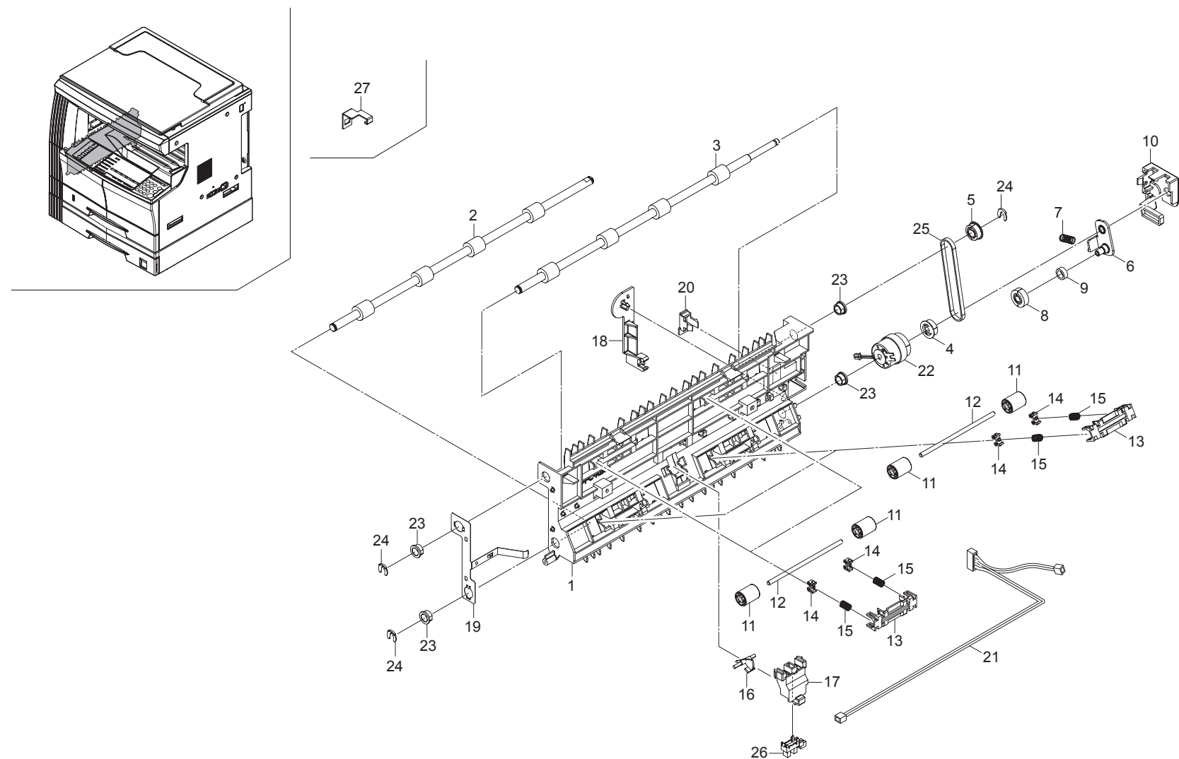
FIG. 18 Option III (DU-410)
