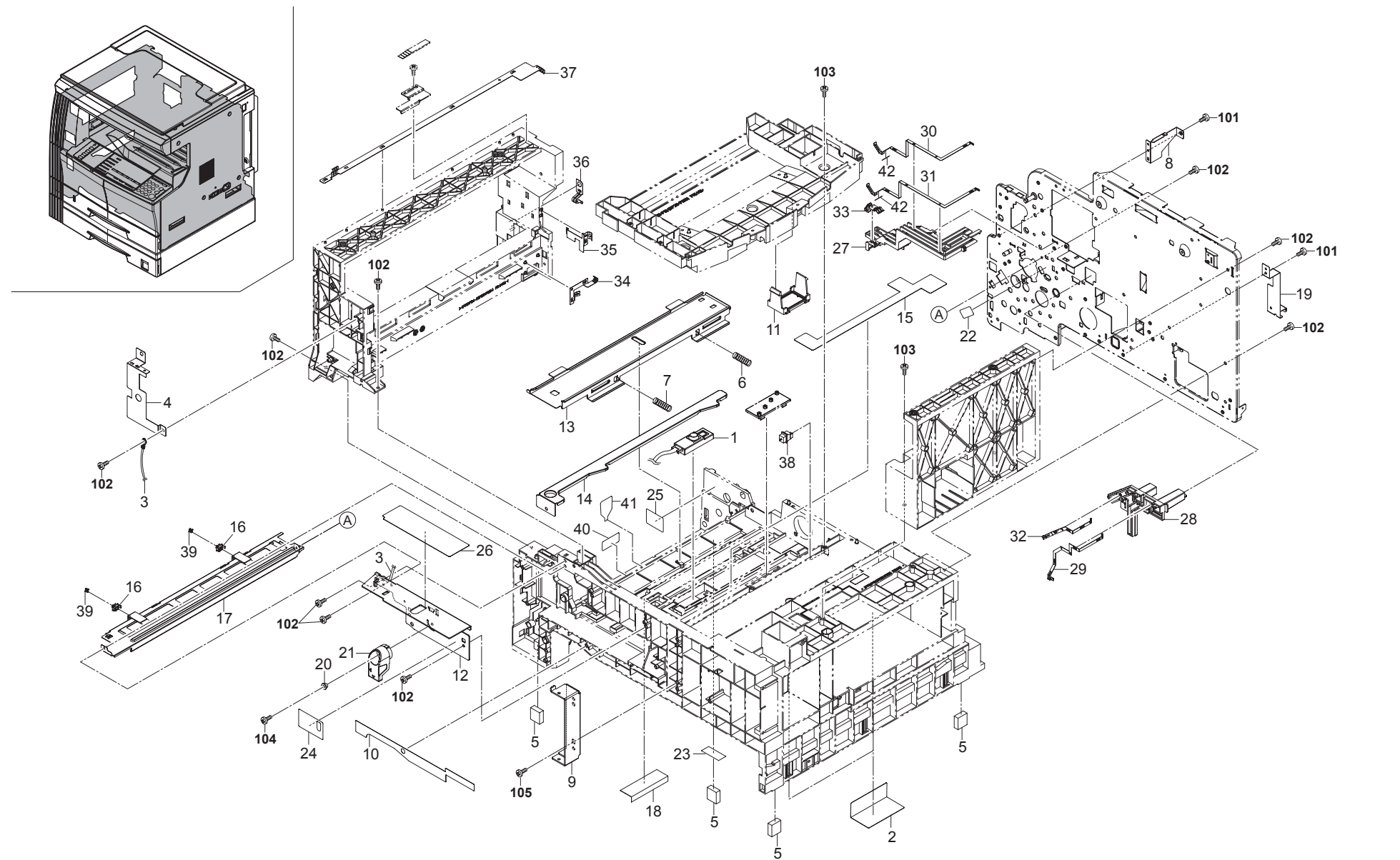
FIG. 2 Frames
