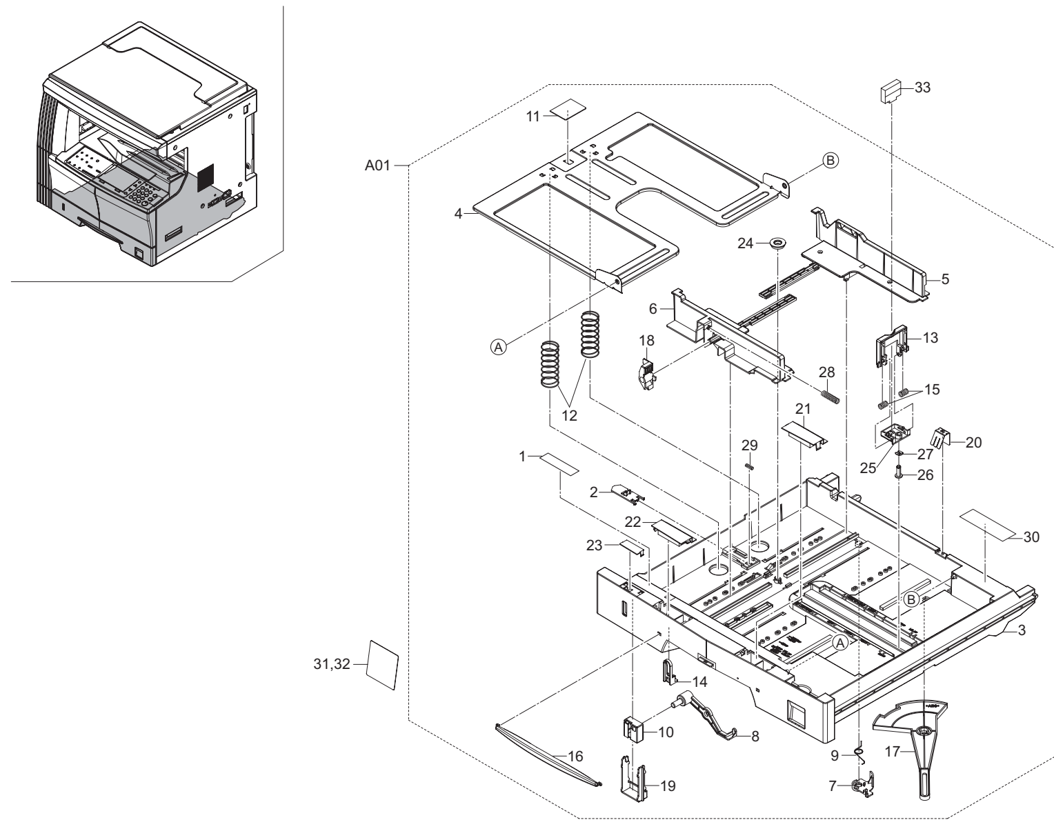
FIG. 3 Cassette
