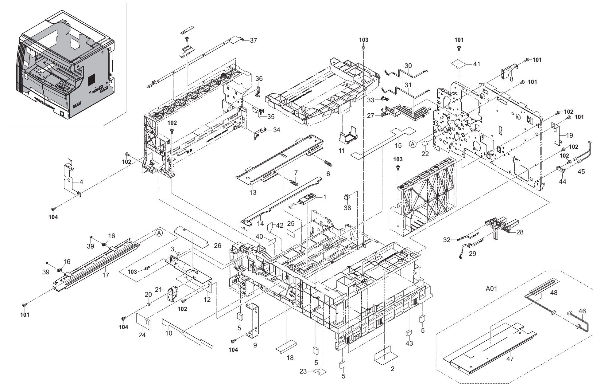
FIG. 2 Frames
