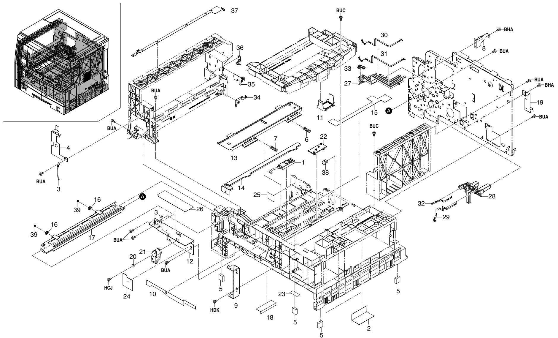
FIG. 2 FRAMES
