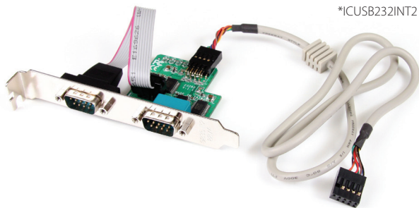
*ICUSB232INT2 shown
