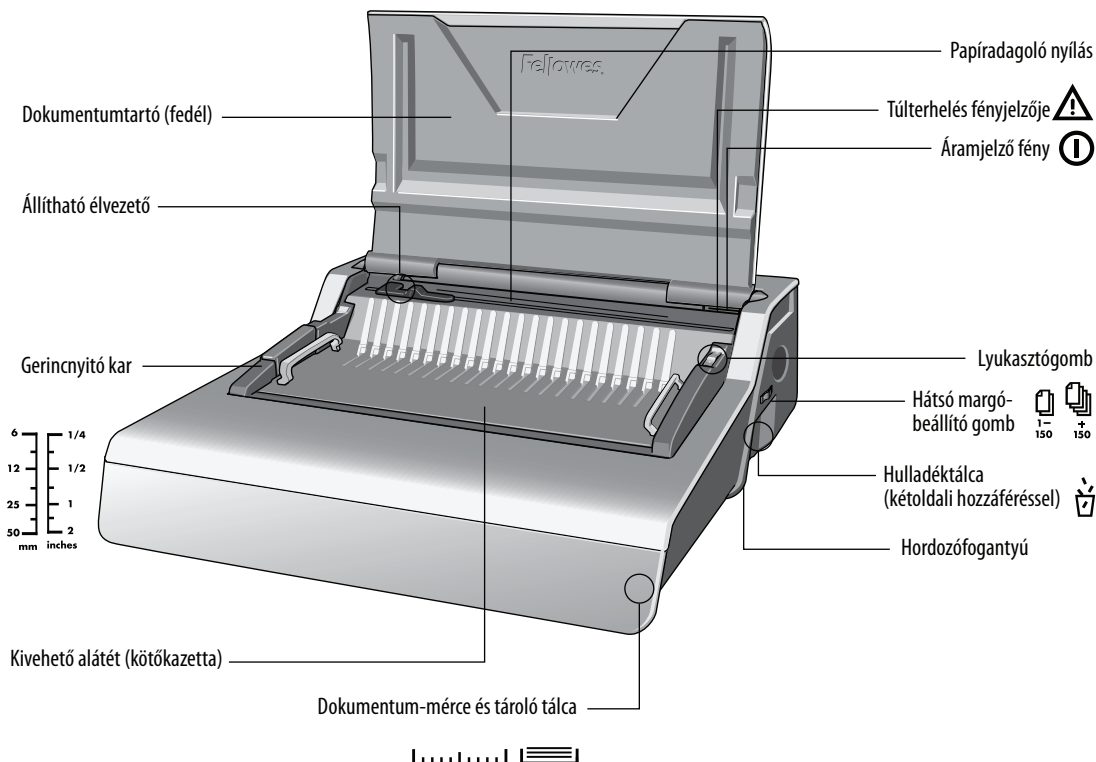
Gerincartó és dokumentum-mérce
