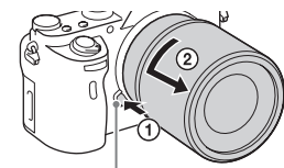
Przycisk zwolnienia obiektywu
