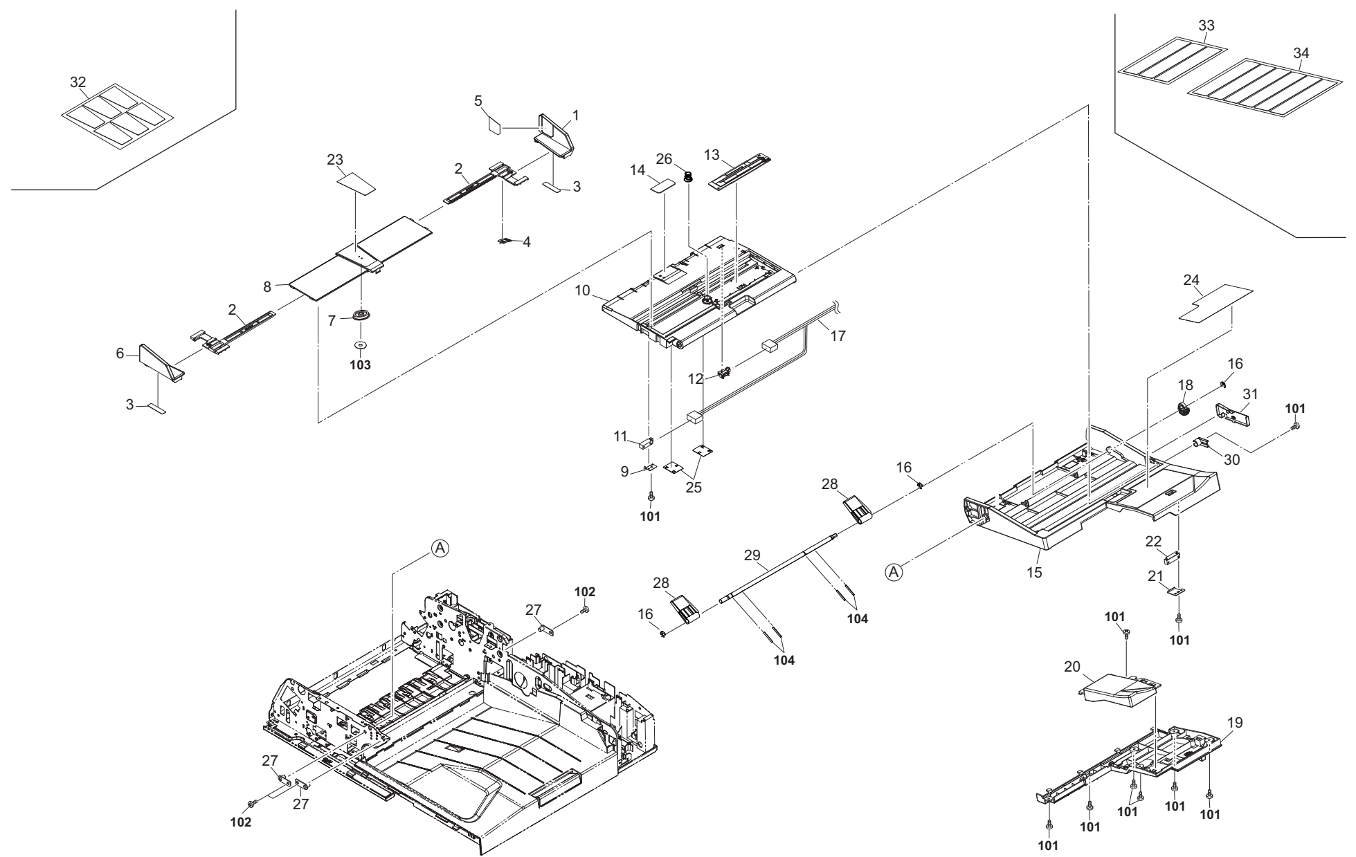
FIG. 38 Table Assy(DP)
