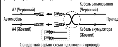
Стандартний варіант схеми підключення проводів
