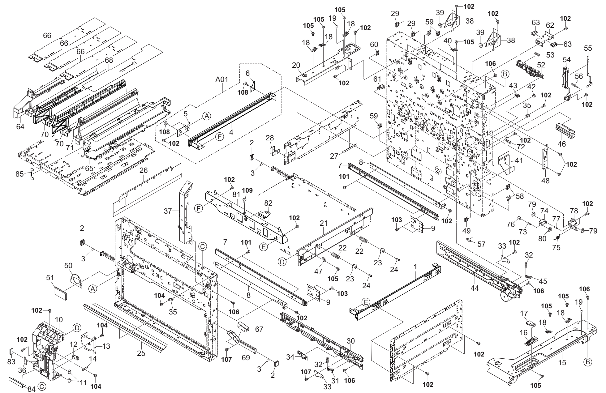
FIG. 4 Frames 1
