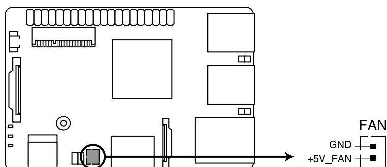
Tinker Board 2 / 2S FAN connector
