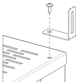
Montage van de wandhouder (optioneel)
