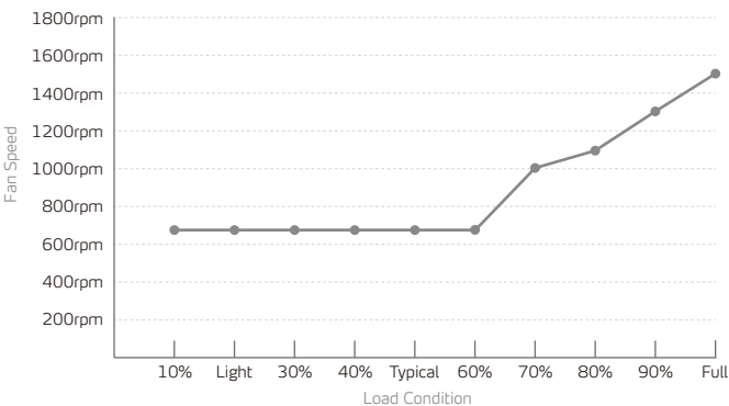
кривая вентилятора блока питания
