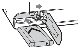
Akkumulátorkioldó kar
