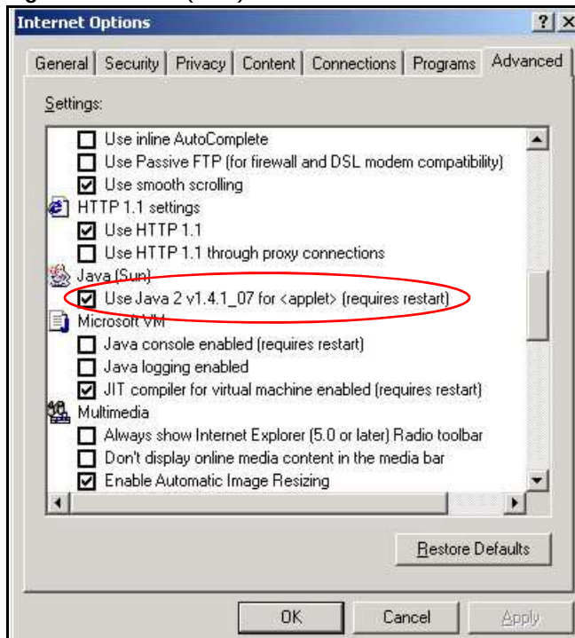
Figure 248 Java (Sun)
