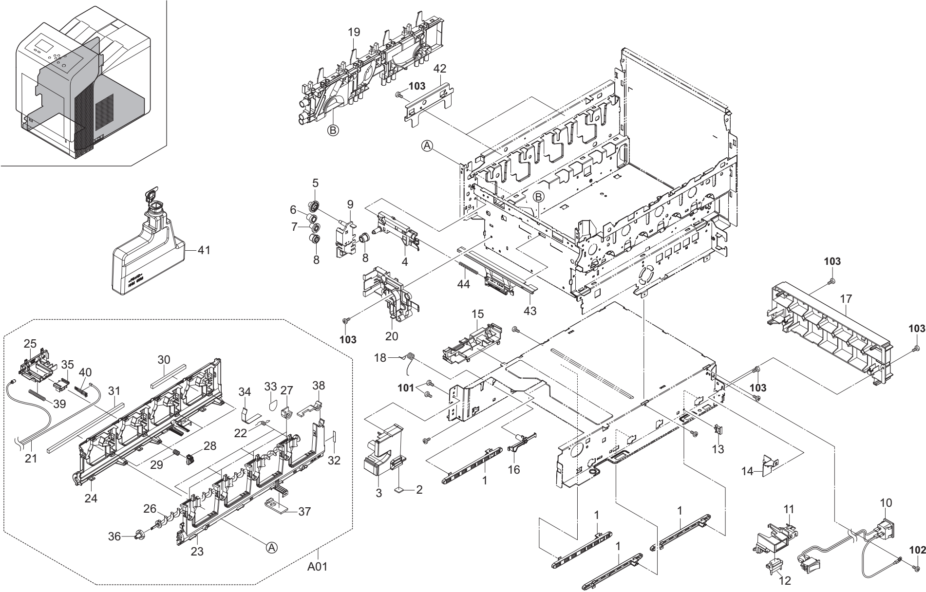
FIG. 4 Frames 2
