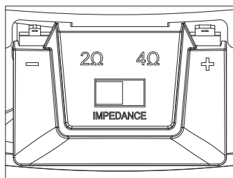
2-ohmsinställning
