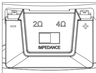
2 Ohm-Einstellung
