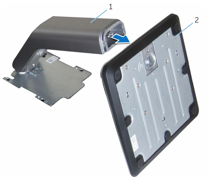
1 stand riser
