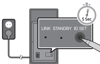
Bassokaiuttimen takaosa
