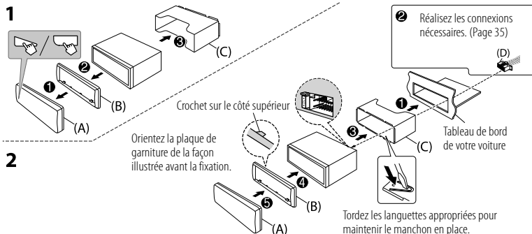
(B) Plaque d'assemblage (×1)
