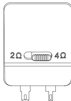
Réglage 4 ohms
